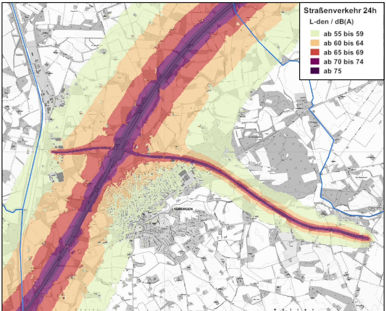
Karte 1: Isophonenkarte Tag L_{den} für Ladbergen, genordet, ohne Maßstab (Auszug aus Anlage 2)
