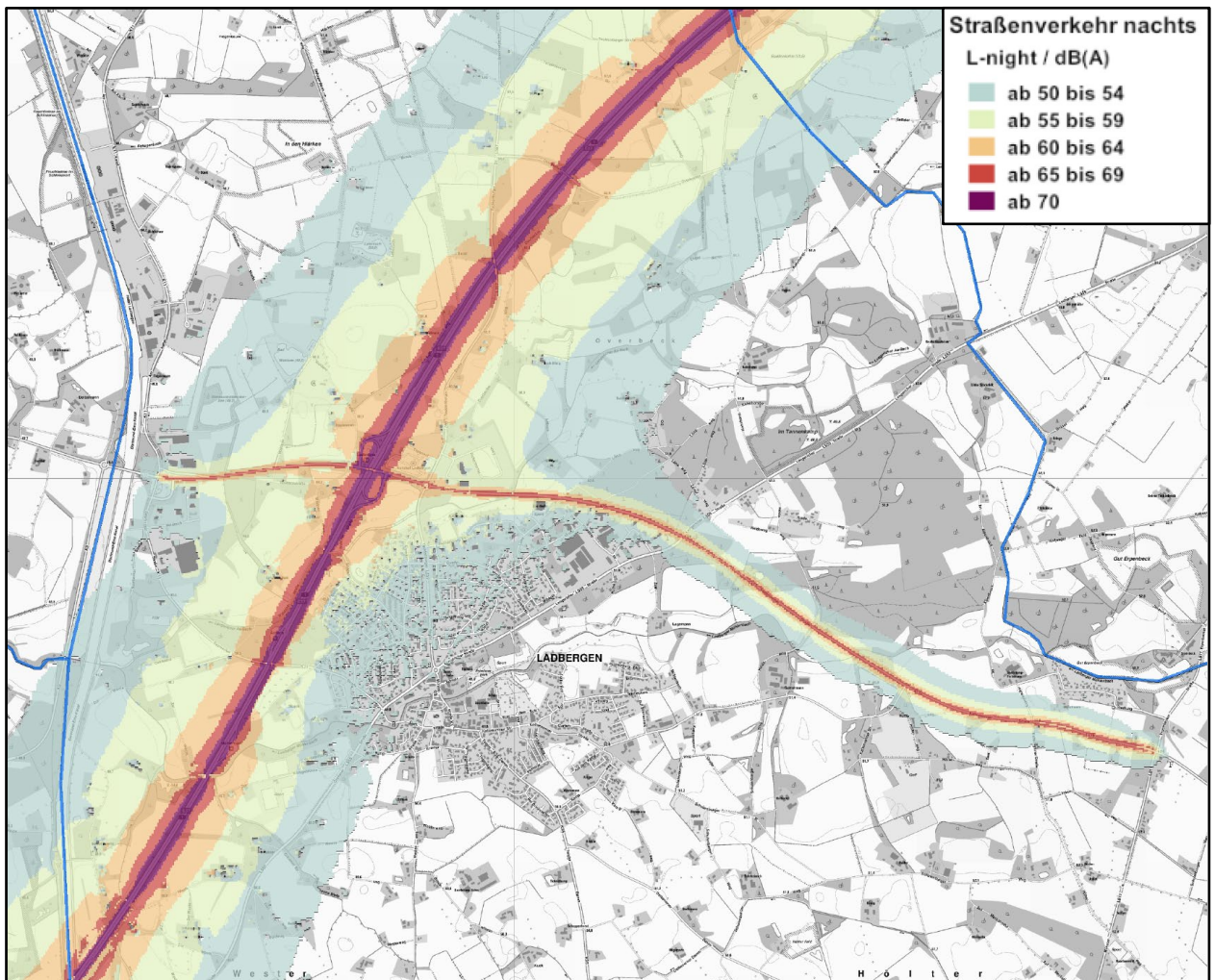
Karte 2: Isophonenkarte Nacht L_{\text{night}} für Ladbergen, genordet, ohne Maßstab (Auszug aus Anlage 3)
